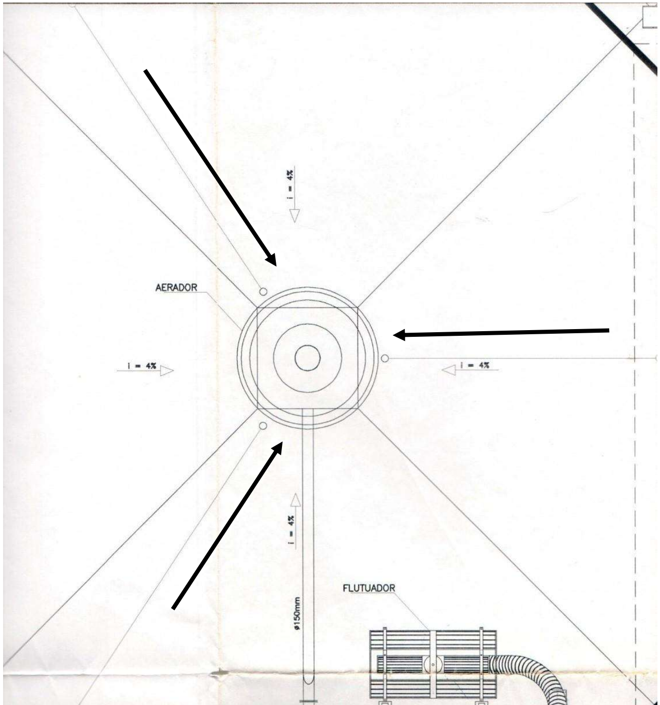
Figura 1: Desenho representando posicionamento do aerador flutuante no centro do tanque com ancoragem através de três pontos.
